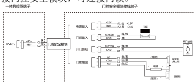
图 4-3 外接门控安全模块
