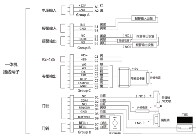
图 4-2 外接设备接线图
