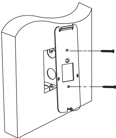
图 5-2 安装挂板
