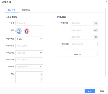
图 8-2 添加人员
