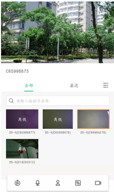
图 8-8 预览界面
