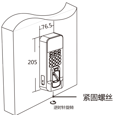
图 5-3 固定设备
