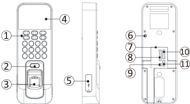
图 3-1 设备外观
