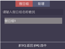
图 7-27 假日组列表
