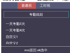
图 7-16 普通班页面
