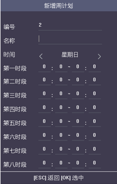
图 7-31 新增周计划
