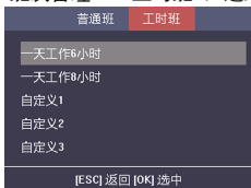
图 7-17 工时班页面
